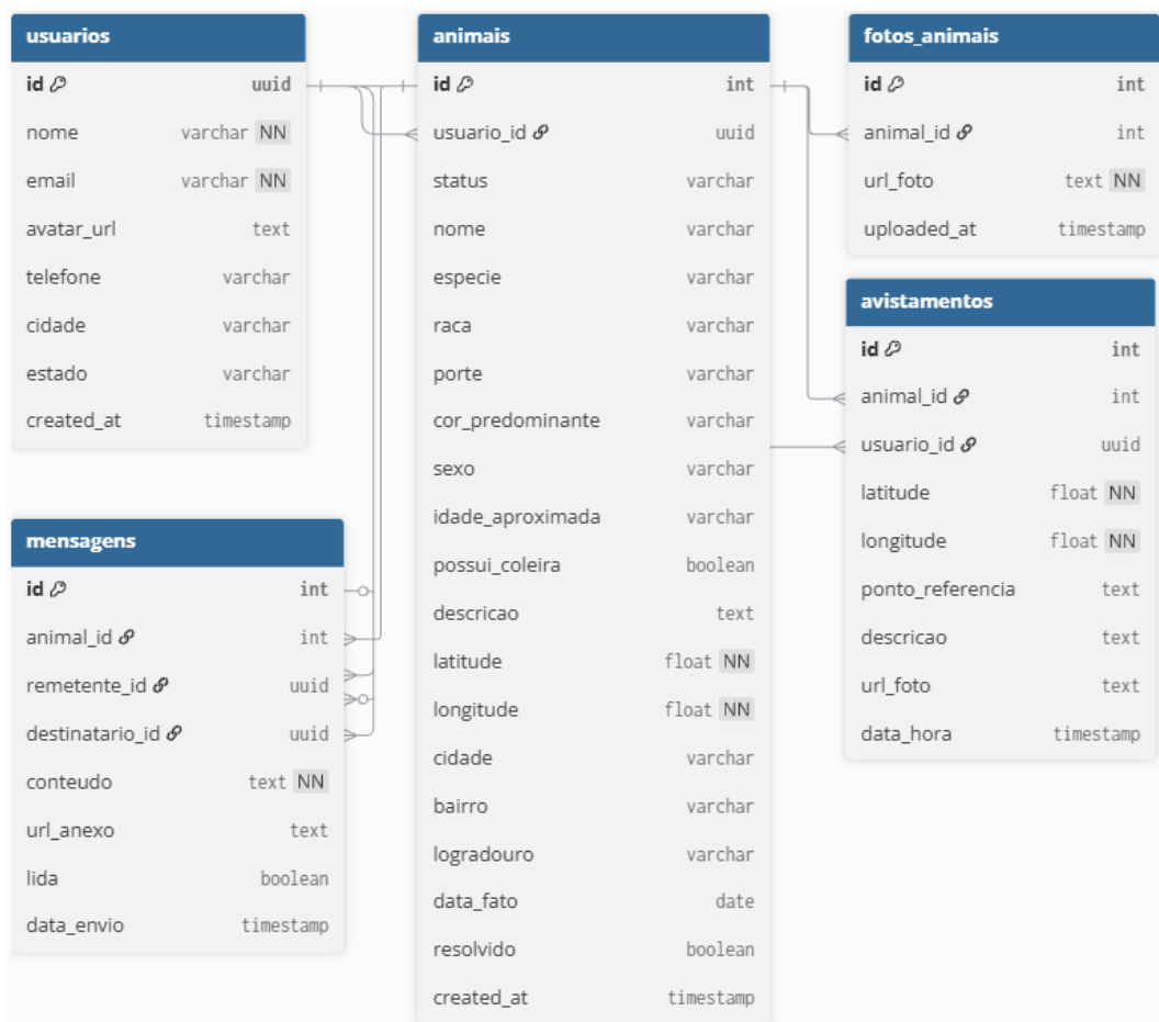
Figura 9: Modelo Lógico Relacional do Banco de Dados PostgreSQL
